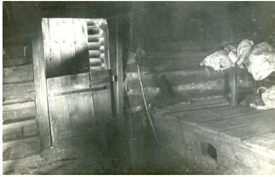
Фото 13. Дверь и кершпель в курной избе, эрзя-мордовское с. Дракино Беднодемьяновского уезда Пензенской губернии. Фото из фотоальбома Н. И. Спрыгиной // МРОКМ КП 3363 Мордва Пензенской губернии. По снимкам Государственного Пензенского областного музея 1923–1928 гг.
