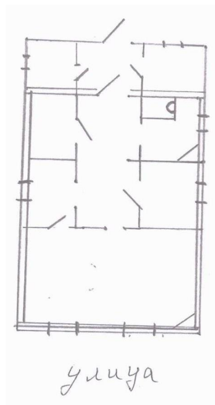
Рис. 3. Планировка эрзя-мордовского дома. Слева – построенного в советское время, справа – в начале XXI в. // ПМА – июль 2021 г., эрзя-мордовская д. Ташто Кшуманця Большеигнатовского района РМ (схемы автора).
