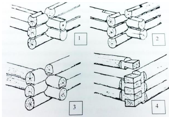
Рис. 1. Способы рубки угла и соединения бревен сруба: 1, 2, 3 – «в чашу», «в угол», 4 – «в лапу» (из кн.: Вавилин В. Ф. Мордовское народное зодчество. Саранск, 1980. С. 46).
